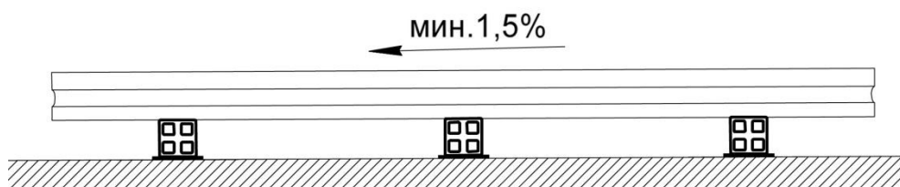
Рис. 2. Пример укладки опорных лаг для обеспечения отвода воды с поверхности профиля
