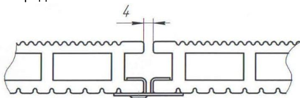
Рис. 6 Продольные стыки
